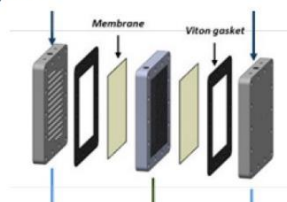
Fig. 5 – Representação gráfica do processo de adsorção e tecnologia de membrana desenvolvido pelo projeto KET4-FGAS
