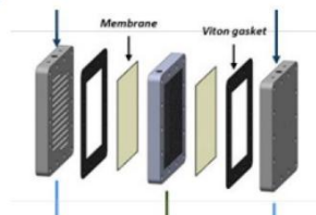
Fig. 5 – Representação gráfica do processo de adsorção e tecnologia de membrana desenvolvido pelo projeto KET4-FGAS
